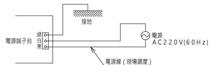
接線圖
